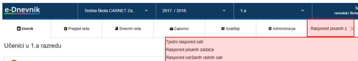
Slika 72 Pretraživanje
