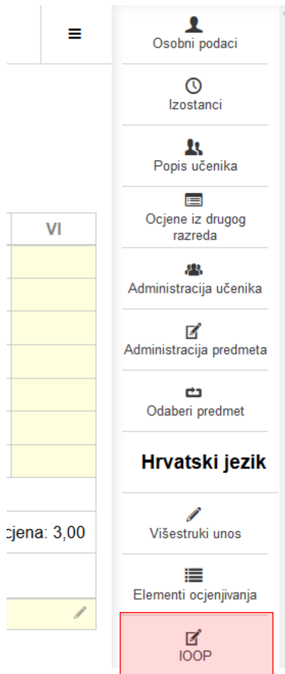
Slika 37 Unos IOOP-a
